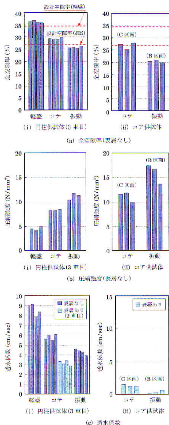
図-4 打設したポーラスコンクリートの各特性と締固め方法の関係
