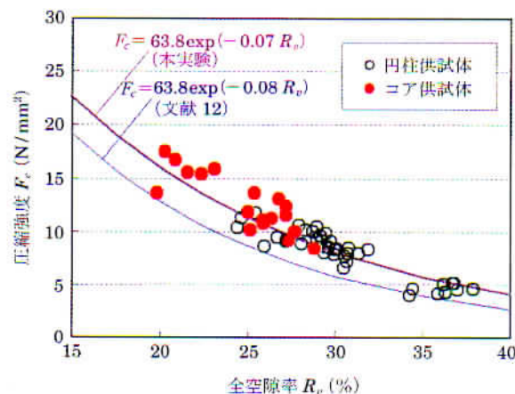
図-5 圧縮強度と全空隙率の関係
