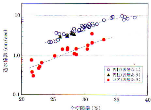
図-6 透水係数と全空隙率の関係
